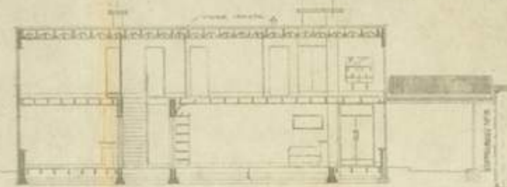
Profiel A-B
